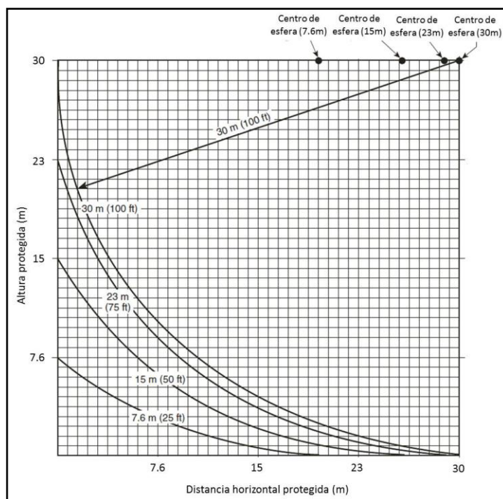
Zona de Protección (Método de Esfera Rodante)
